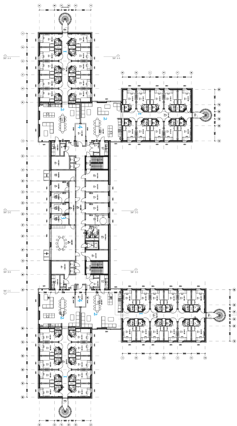
تصویر ۳-۵: بخشی از پلان زندان هالدين
