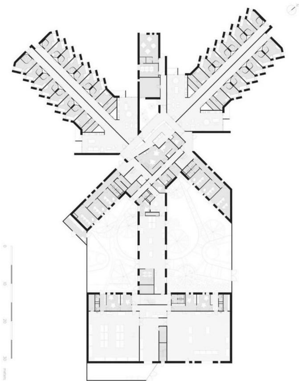
تصویر ۵-۱۶: بخشی از پلان زندان استورستروم
