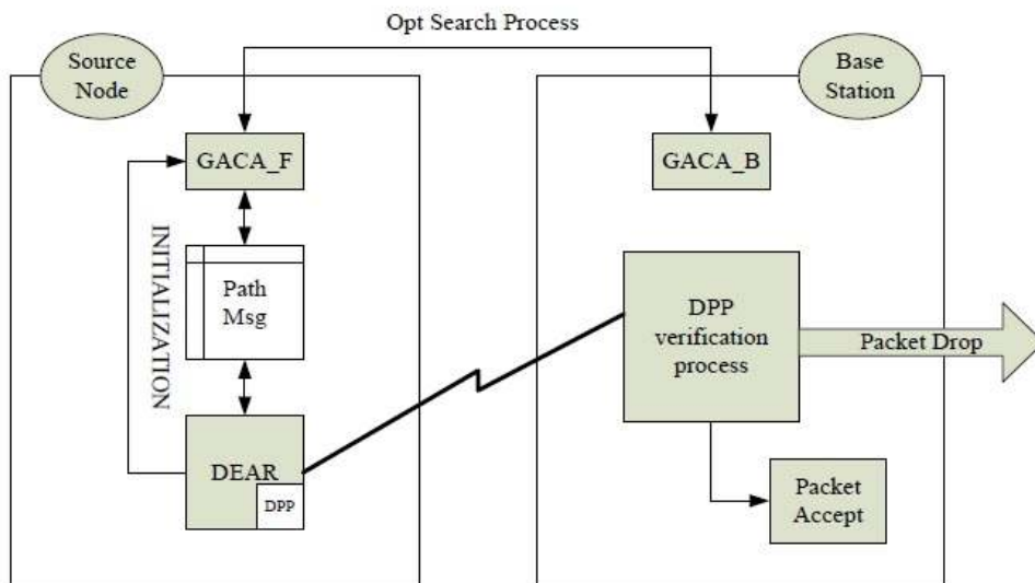
شکل ۲-۱۱ روند اجرای الگوریتم GACA [29]
