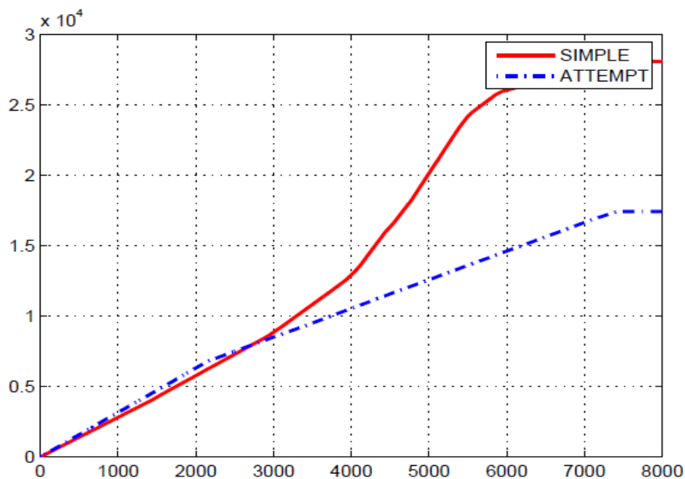
شکل ۲-۶ تجزیه و تحلیل توان عملیاتی پروتکل SIMPLE [20]
