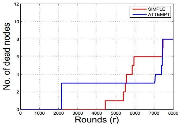
شکل ۷-۲ تجزیه و تحلیل طول عمر شبکه پروتکل SIMPLE [20]
