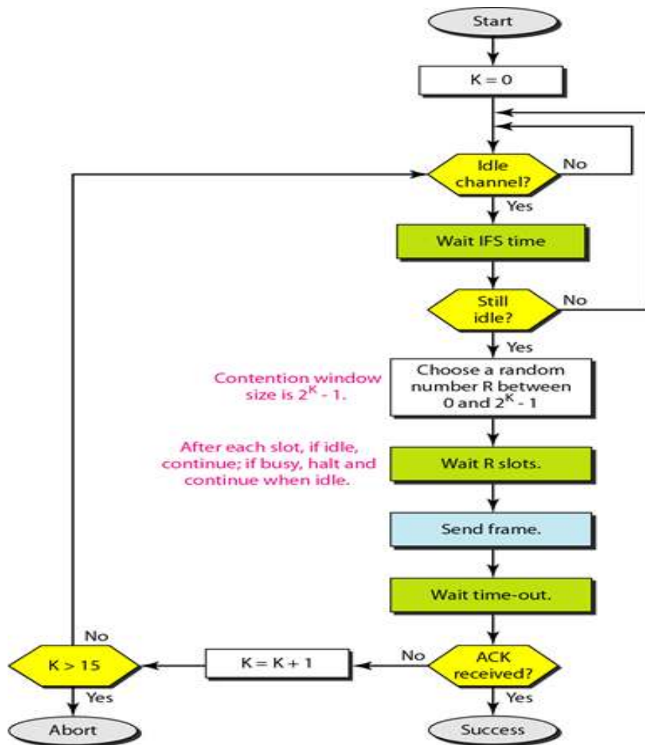
شکل ۲-۱۳ روند اجرایی زمانبند CSMA/CA [31]
