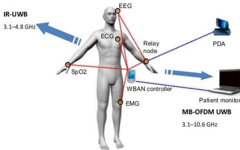
شکل ۲-۳ تکنولوژی UWB در شبکه‌های بی‌سیم ناحیه بدن [15]
