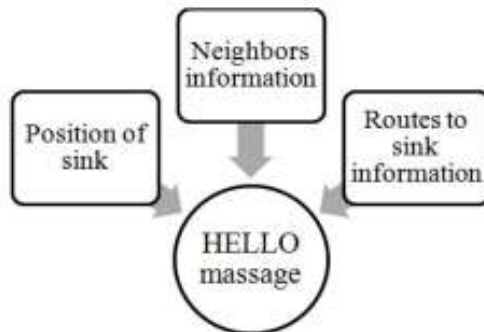
شکل ۲-۸ پیام خوش آمدگویی گره چاهک در پروتکل FEEL [22]
