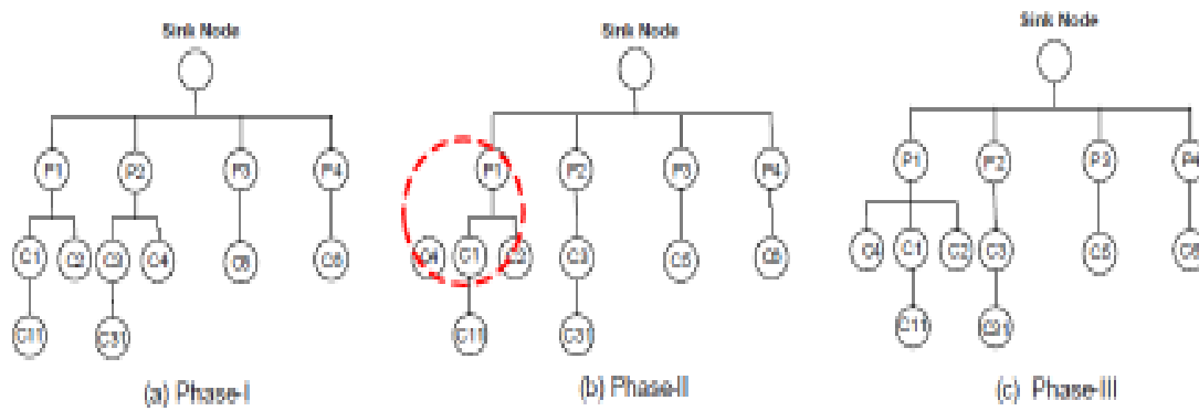
شکل ۲-۴ مراحل اجرایی پروتکل M-ATTEMPT [19]
