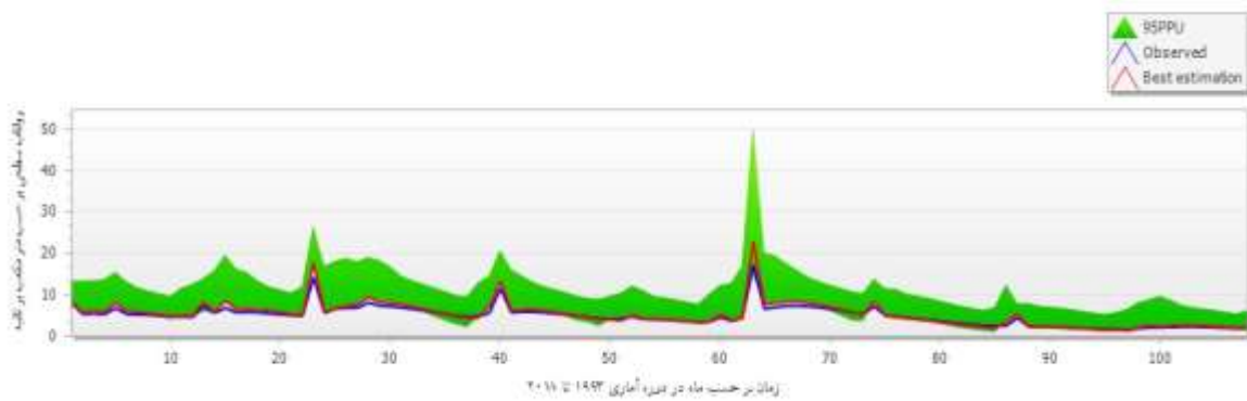
شکل (۶): نتایج صحت‌سنجی مدل SWAT با استفاده از الگوریتم SUFI-2 برای شبیه‌سازی رواناب در ایستگاه هیدرومتری آفرینه Figure (6): SWAT Model Validation Results Using SUFI-2 Algorithm for Simulation of Runoff at Afarineh Hydrometric Station
