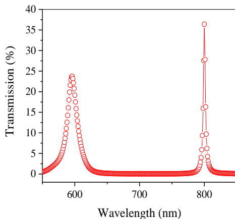
شکل ۸: طیف عبوری از بلور نوری [\text{Si/SiO}_2]^3/\text{TiO}_2/[\text{Si/SiO}_2]^3/\text{Si}_3\text{N}_4 در طول موج کاری ترکیبی ۶۰۰ و ۸۰۰ نانومتر.
