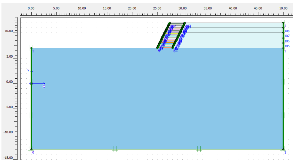
شکل ۴-۱: نمای کلی از مدل شیروانی و پی آن در نرم افزار به همراه لایه‌های افقی ژئوسل در قسمت نما
