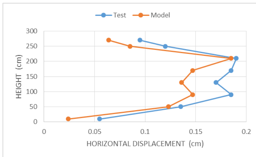
شکل ۳-۹: مقایسه تغییرمکان افقی در آزمایش و مدل‌سازی
