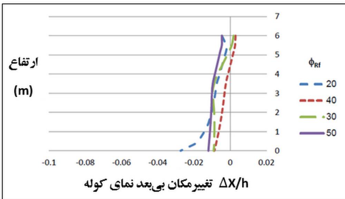
شکل ۲-۱۱: جابه‌جایی دیوار در ارتفاع (عنایتی و قضاوی، ۱۳۹۳) [5]
