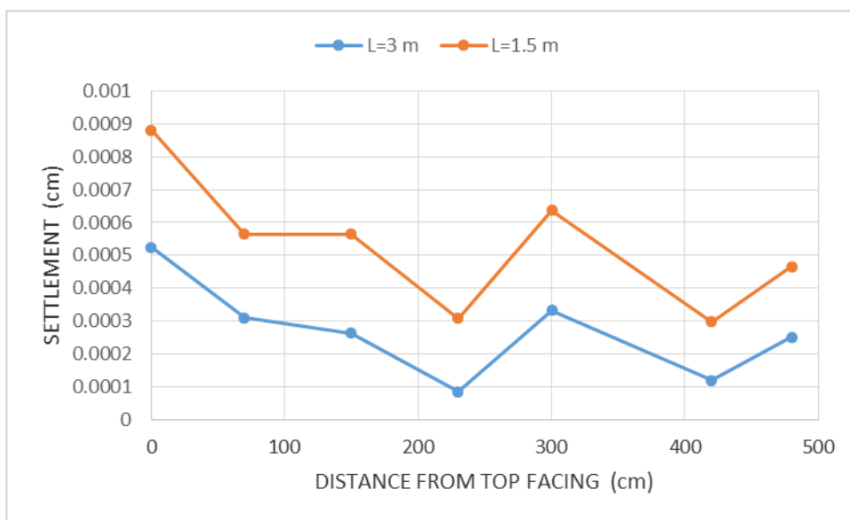
۲۷-۴: مقایسه نشست شیروانی برای دو مدل مسلح شده در نما با لایه‌های مسلح کننده به طول ۳ و ۱/۵ متر (سلول‌های ژئوسل پر شده با خاک ماسه و ژئوسل با M=500 \text{ kN/m} )
