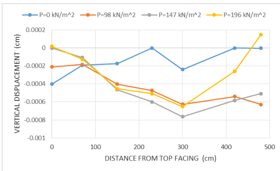
۴-۴۵: مقایسه نشست شیروانی نما برای مدل‌های مسلح شده در نما با لایه ژئوسل به طول ۳ متر و با M=500 \text{ kN/m} و پر شده با خاک شن (تأثیر سربار)
