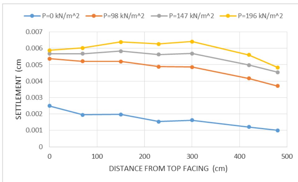
۴-۴۷: مقایسه نشست شیروانی برای مدل‌های مسلح شده در نما با لایه ژئوسل به طول ۳ متر در نما و ۵ متر در عمق و با M=200 \text{ kN/m} و پر شده با خاک ماسه (تأثیر سربار)
