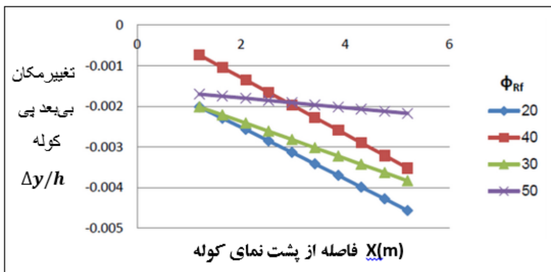
شکل ۲-۱۰: تغییرات تغییرمکان پی دیوار کوله به نسبت فاصله از دیوار (عنایتی و قضاوی، ۱۳۹۳)
