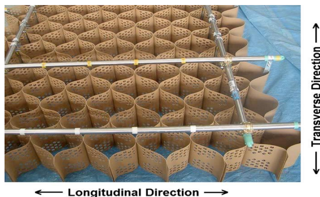
شکل ۳-۴: نمونه ژئوسل‌های مورد استفاده در آزمایش لینگ و همکاران (۲۰۰۹) [17]
