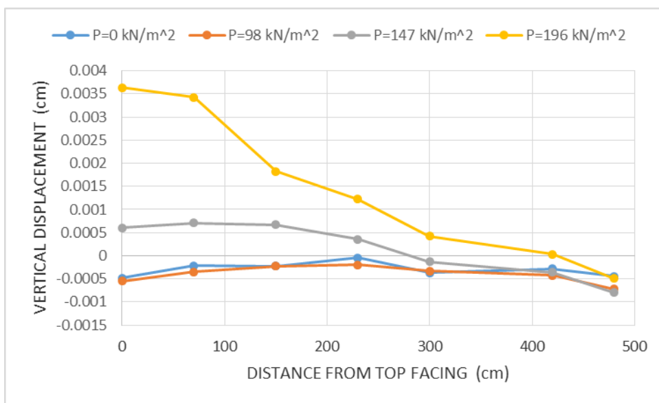
۶۱-۴: مقایسه نشست شیروانی برای مدل‌های مسلح شده در نما با لایه ژئوسل به طول ۱/۵ متر و با M=500 \text{ kN/m} و پر شده با خاک شن (تأثیر سربار)
