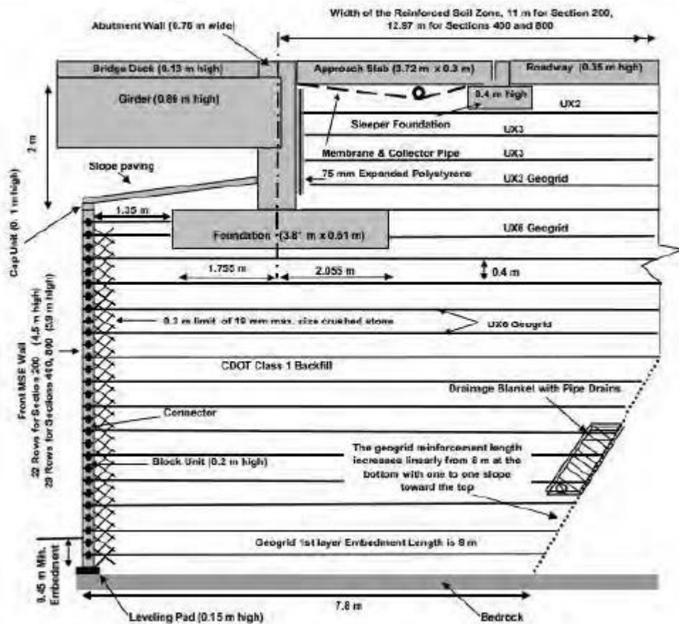
شکل ۲-۹: مقطع کوله مسلح، پروژه فاندر (عنایتی و قضاوی ۱۳۹۳) [5]
