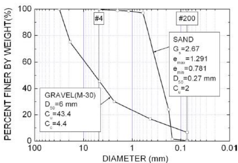
شکل ۳-۳: نتایج آزمایش دانه‌بندی خاک‌های ماسه‌ای و شنی لینگ و همکاران (۲۰۰۹) [17]
