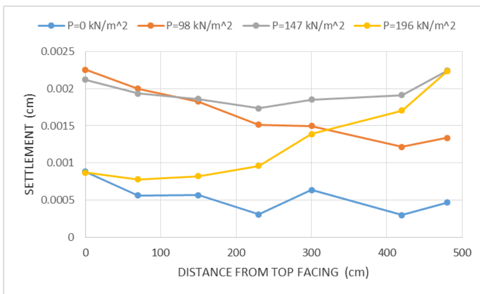
۵۹-۴: مقایسه نشست شیروانی برای مدل‌های مسلح شده در نما با لایه ژئوسل به طول ۱/۵ متر و با M=500 \text{ kN/m} و پر شده با خاک ماسه (تأثیر سربار)
