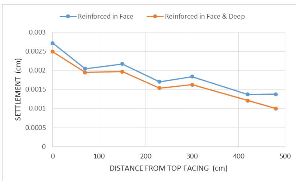
۴-۱۵: مقایسه نشست شیروانی برای دو مدل مسلح شده در نما و مسلح شده در عمق و نما (سلول‌های ژئوسل پر شده با خاک ماسه ای و ژئوسل با M=200 \text{ kN/m} )
