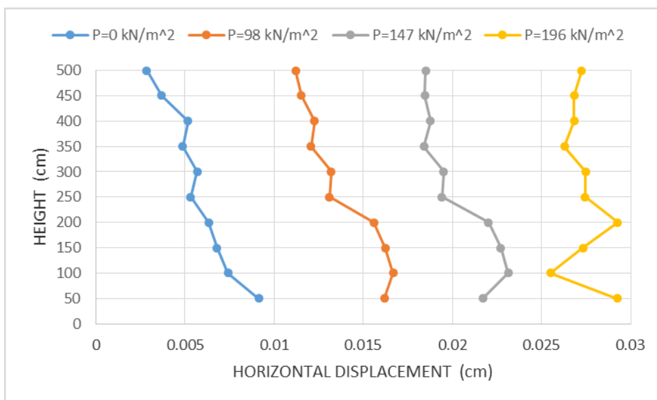
۴-۴۶: مقایسه تغییر مکان افقی نما برای مدل‌های مسلح شده در نما با لایه ژئوسل به طول ۳ متر در نما و ۵ متر در عمق و با M=200 \text{ kN/m} و پر شده با خاک ماسه (تأثیر سربار)
