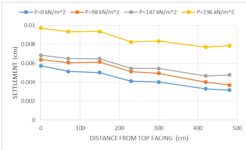
۵۵-۴: مقایسه نشست شیروانی برای مدل‌های مسلح شده در نما با لایه ژئوسل به طول ۱/۵ متر و با M=200 \text{ kN/m} و پر شده با خاک ماسه (تأثیر سربار)
