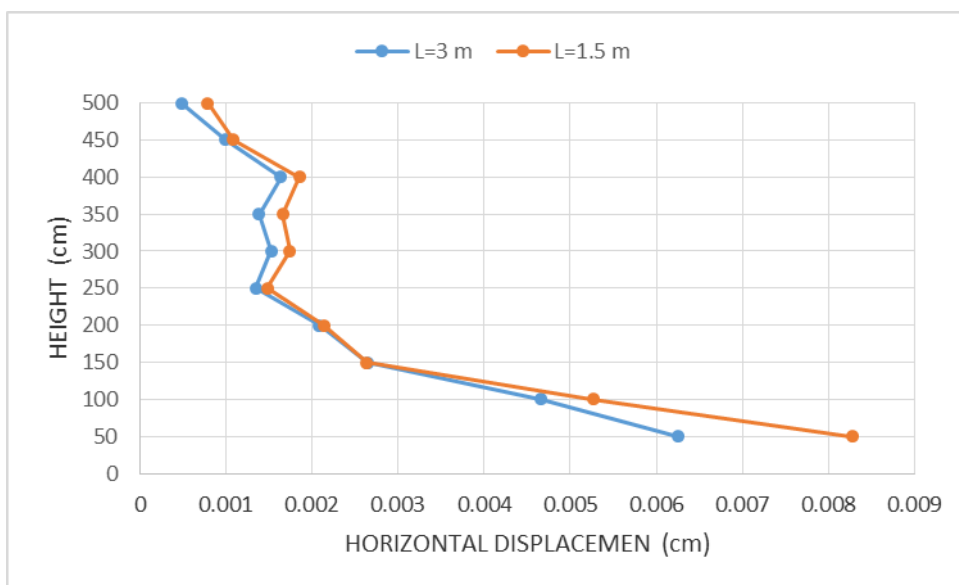
۲۸-۴: مقایسه تغییر مکان افقی نما برای دو مدل مسلح شده در نما با لایه‌های مسلح کننده به طول ۳ و ۱/۵ متر (سلول‌های ژئوسل پر شده با خاک شن و ژئوسل با M=500 \text{ kN/m} )
