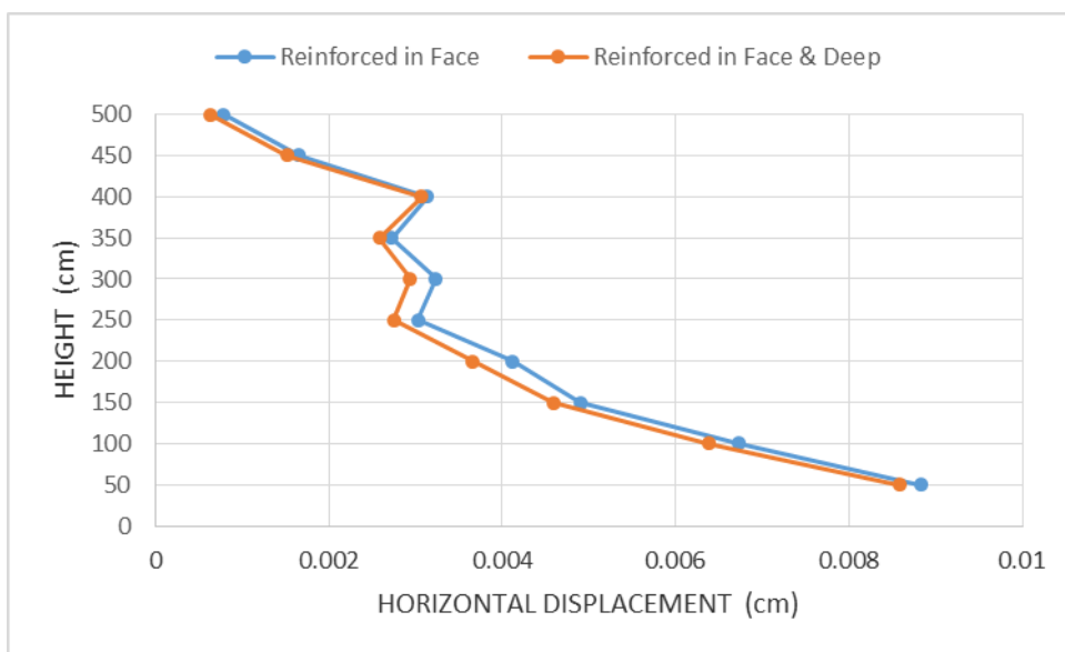
۴-۱۶: مقایسه تغییر مکان افقی نما برای دو مدل مسلح شده در نما و مسلح شده در عمق و نما (سلول‌های ژئوسل پر شده با خاک شن و ژئوسل با M=200 \text{ kN/m} )
