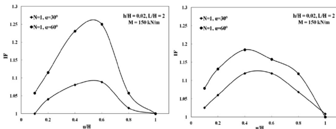
شکل ۲-۱۳: ضریب بهبود عملکرد برای خاک‌های ماسه‌ای و رسی در پژوهش مهدی پور و همکاران
