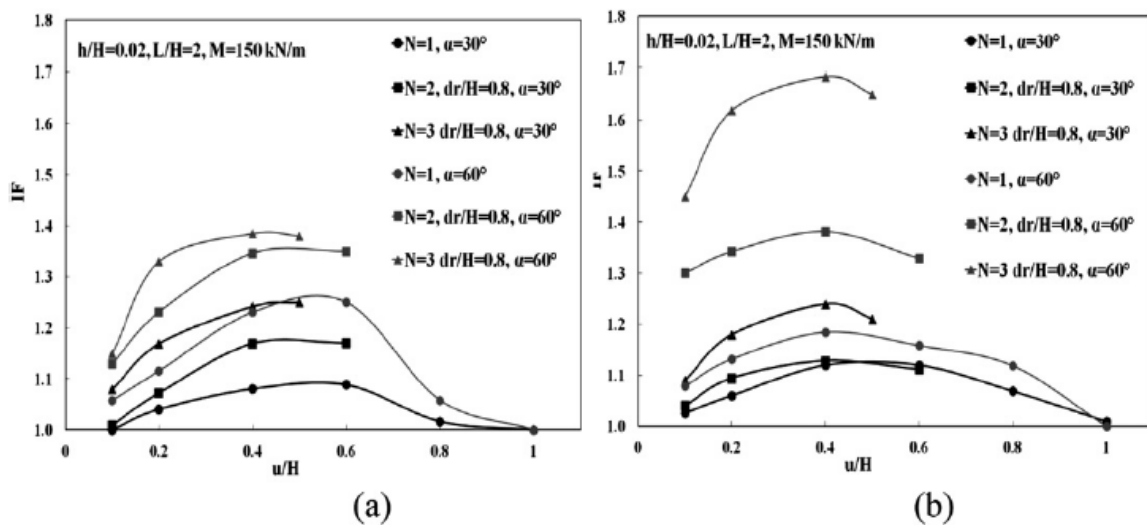
شکل ۲-۱۶: تأثیر تعداد لایه مسلح کننده در پایداری شیروانی (a) برای خاک ماسه‌ای و (b) برای خاک رسی در پژوهش مهدی پور و همکاران (۲۰۱۳) [15]
