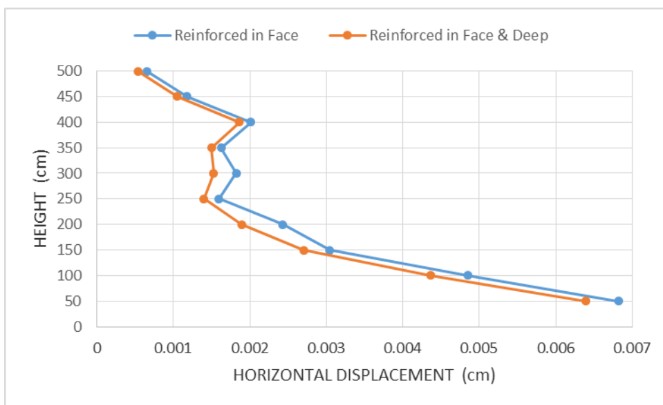
۴-۱۸: مقایسه تغییر مکان افقی نما برای دو مدل مسلح شده در نما و مسلح شده در عمق و نما (سلول‌های ژئوسل پر شده با خاک ماسه و ژئوسل با M=500 \text{ kN/m} )
