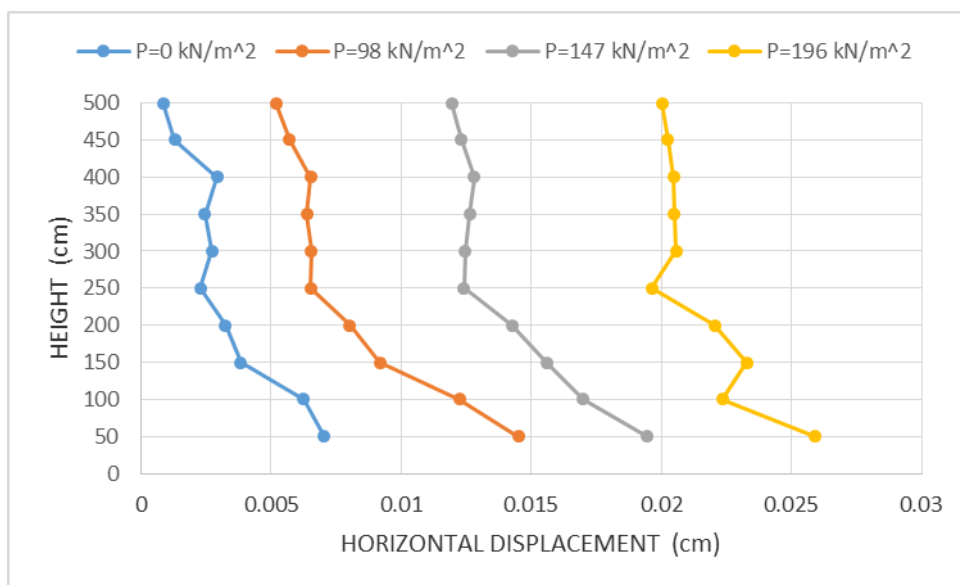
۴-۵۸: مقایسه تغییر مکان افقی نما برای مدل‌های مسلح شده در نما با لایه ژئوسل به طول ۱/۵ متر و با M=500 \text{ kN/m} و پر شده با خاک ماسه (تأثیر سربار)
