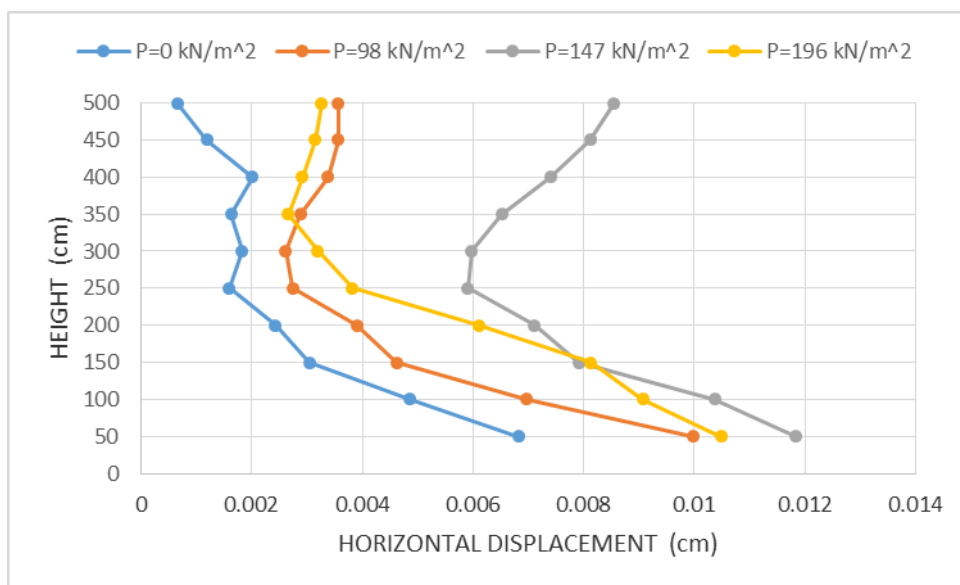
۴-۴۲: مقایسه تغییر مکان افقی نما برای مدل‌های مسلح شده در نما با لایه ژئوسل به طول ۳ متر و با M=500 \text{ kN/m} و پر شده با خاک ماسه (تأثیر سربار)
