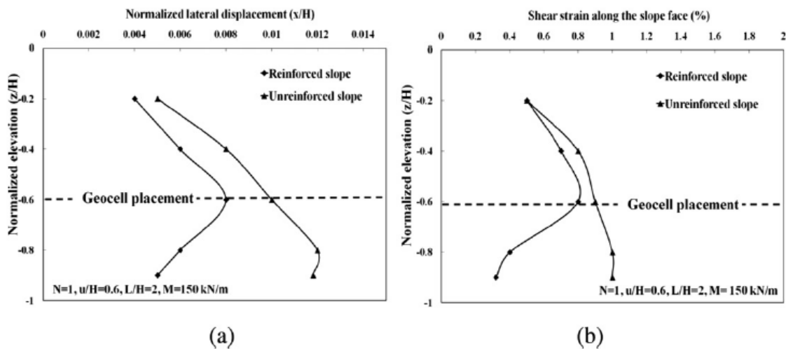
شکل ۲-۱۵: تغییرمکان جانبی شیروانی ماسه‌ای و نیز کرنش برشی در نمای آن در تحقیق مهدی پور و همکاران (۲۰۱۳) [15]
