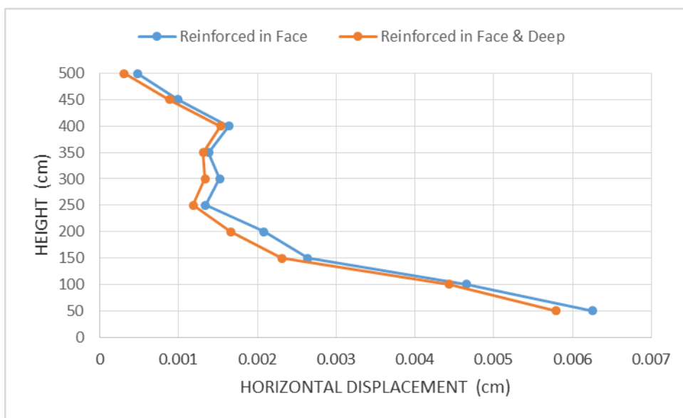
۲۰-۴: مقایسه تغییر مکان افقی نما برای دو مدل مسلح شده در نما و مسلح شده در عمق و نما (سلول‌های ژئوسل پر شده با خاک شن و ژئوسل با M=500 \text{ kN/m} )
