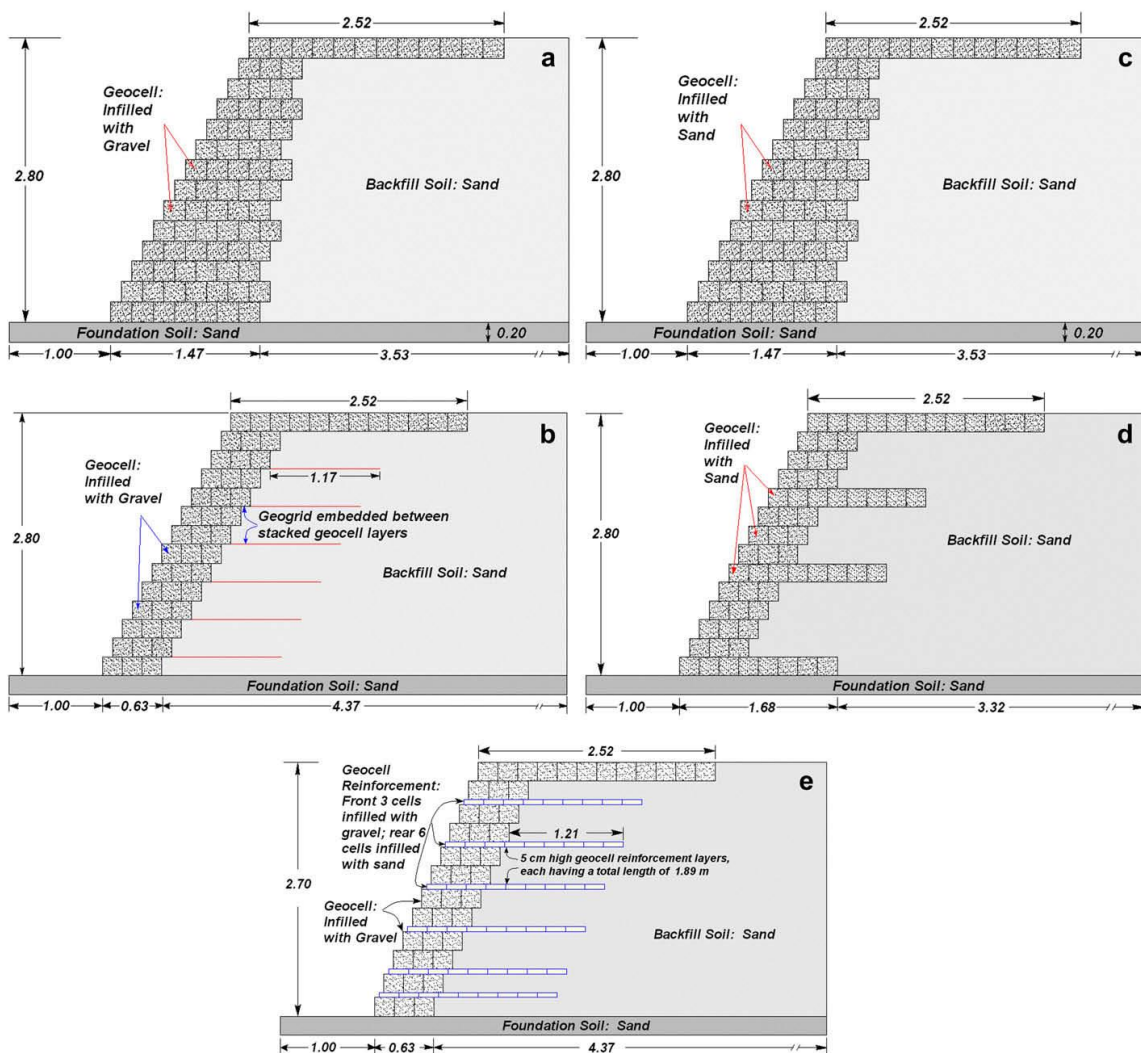
شکل ۲-۲۰: شمای کلی پنج آزمایش لشچینسکی و همکاران در سال (۲۰۰۹) [16]
