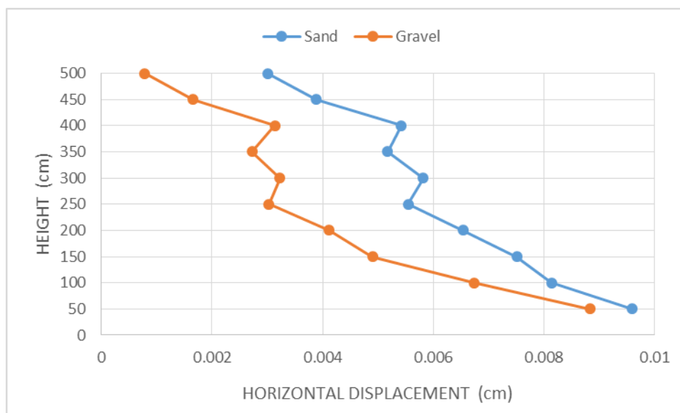
شکل ۴-۷: مقایسه تغییرمکان افقی نما برای دو مدل مسلح (پر شده با ماسه و شن)
