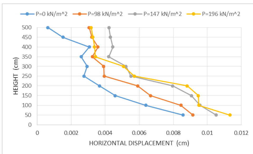
۴-۴۸: مقایسه تغییر مکان افقی نما برای مدل‌های مسلح شده در نما با لایه ژئوسل به طول ۳ متر در نما و ۵ متر در عمق و با M=200 \text{ kN/m} و پر شده با خاک شن (تأثیر سربار)
