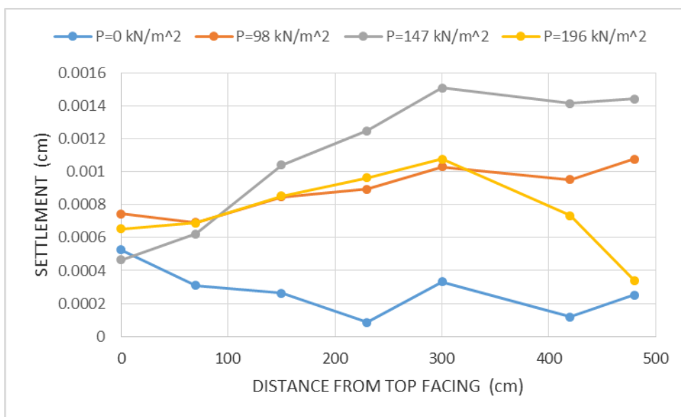
۴-۲۳: مقایسه نشست شیروانی نما برای مدل‌های مسلح شده در نما با لایه ژئوسل به طول ۳ متر و با M=500 \text{ kN/m} و پر شده با خاک ماسه (تأثیر سربار)
