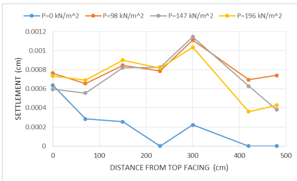
۴-۴۹: مقایسه نشست شیروانی برای مدل‌های مسلح شده در نما با لایه ژئوسل به طول ۳ متر در نما و ۵ متر در عمق و با M=200 \text{ kN/m} و پر شده با خاک شن (تأثیر سربار)
