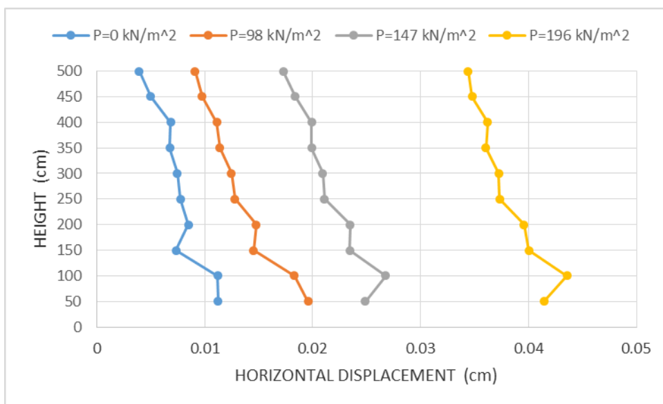
۶۲-۴: مقایسه تغییر مکان افقی نما برای مدل‌های مسلح شده در نما با لایه ژئوسل به طول ۱/۵ متر در نما و ۴ متر در عمق و با M=200 \text{ kN/m} و پر شده با خاک ماسه (تأثیر سربار)
