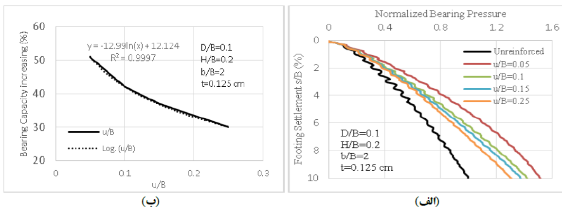
شکل ۲-۴: نتایج مربوط به عمق قرارگیری لایه ژئوسل (غفارپور و شیبانی، ۱۳۹۳) [3]
