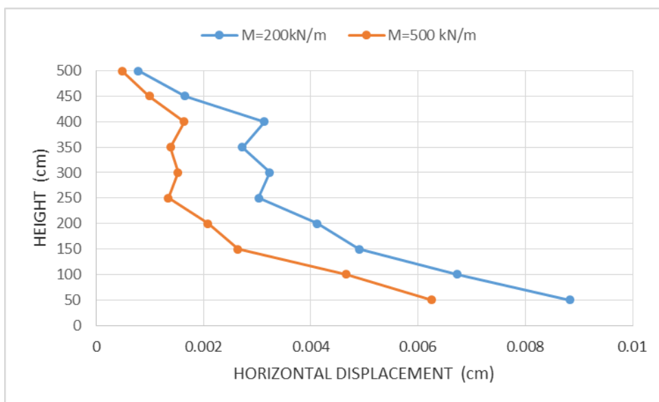
۴-۱۱: مقایسه تغییر مکان افقی نما برای دو مدل مسلح شده با ژئوسل با سختی محوری ۲۰۰ و ۵۰۰ کیلونیوتن برمتر (پوشده با شن)
