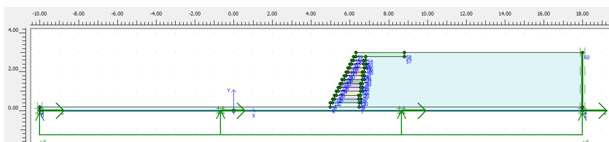
شکل ۳-۵: مدل دیوار مسلح به ژئوسل در نرم‌افزار پلکسیس
