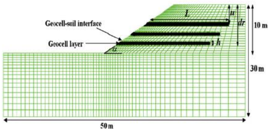
شکل ۲-۱۲: مدل پژوهش مهدی پور و همکاران (۲۰۱۳) [15]
