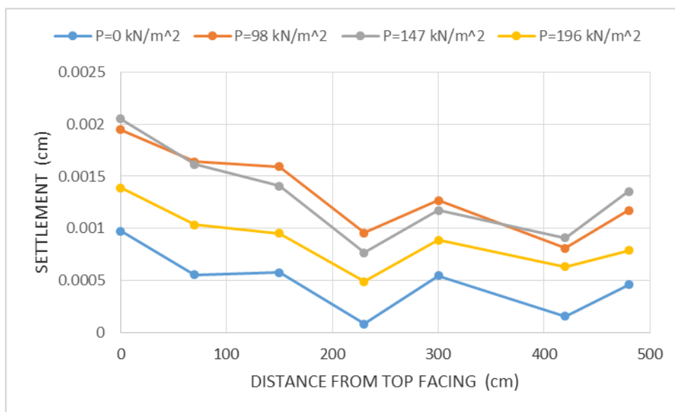
۴-۵۷: مقایسه نشست شیروانی نما برای مدل‌های مسلح شده در نما با لایه ژئوسل به طول ۱/۵ متر و با M=200 \text{ kN/m} و پر شده با خاک شن (تأثیر سربار)
