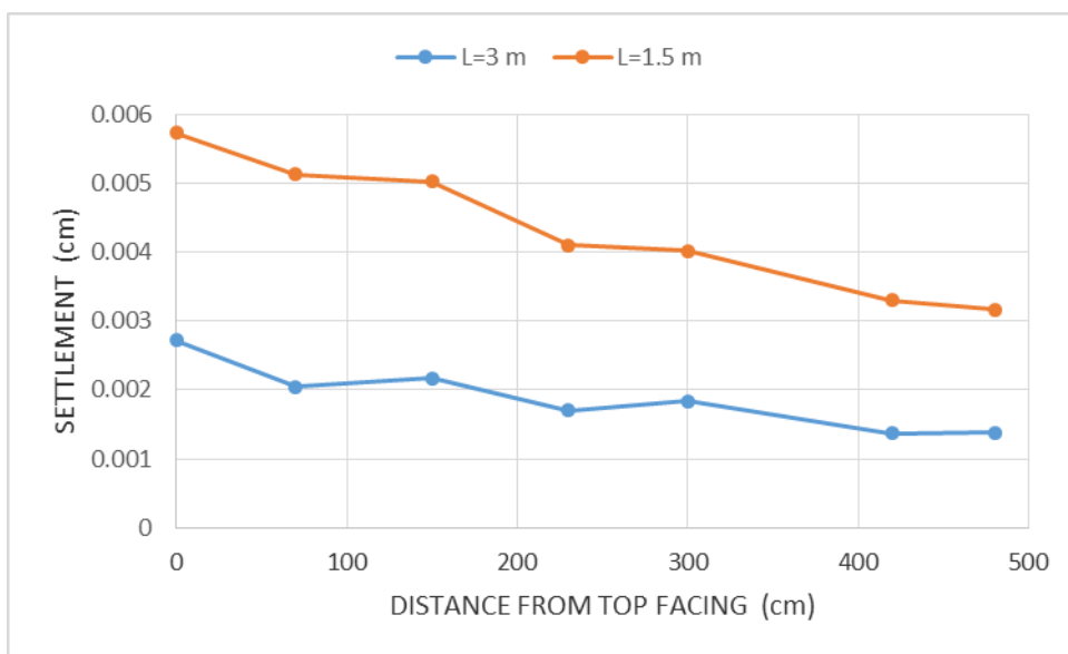
۲۳-۴: مقایسه نشست شیروانی برای دو مدل مسلح شده در نما با لایه‌های مسلح کننده به طول ۳ و ۱/۵ متر (سلول‌های ژئوسل پر شده با خاک ماسه و ژئوسل با M=200 \text{ kN/m} )
