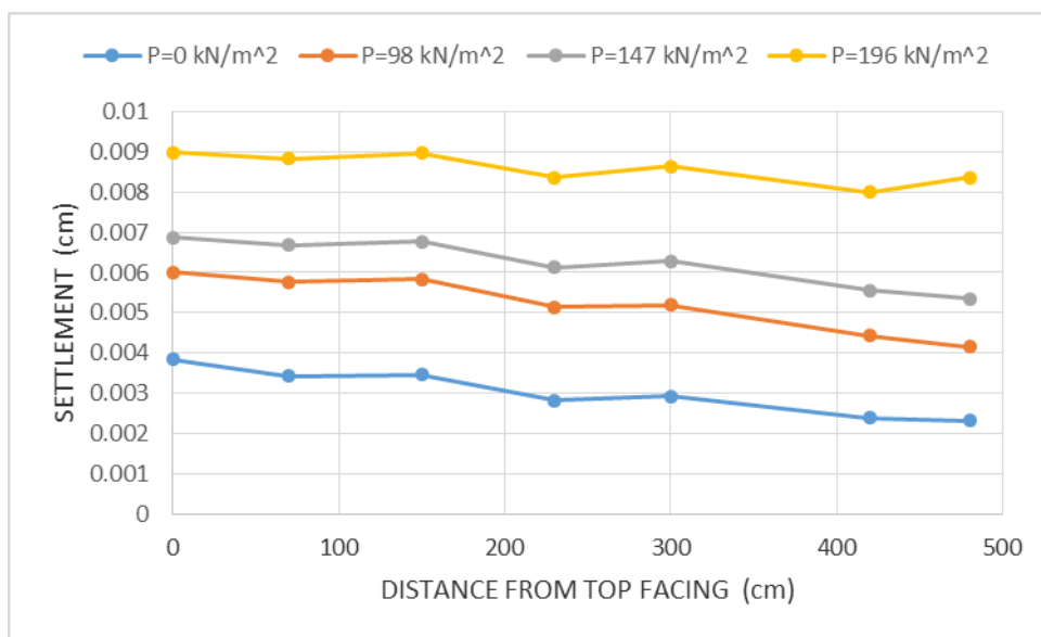
۶۳-۴: مقایسه نشست شیروانی برای مدل‌های مسلح شده در نما با لایه ژئوسل به طول ۱/۵ متر در نما و ۴ متر در عمق و با M=200 \text{ kN/m} و پر شده با خاک ماسه (تأثیر سربار)
