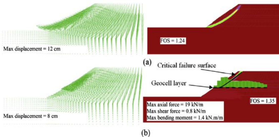
شکل ۲-۱۴: سطوح گسیختگی و بردارهای تغییرمکان برای خاک‌های دانه‌ای و رسی در تحقیق مهدی پور و همکاران (۲۰۱۳) [15]
