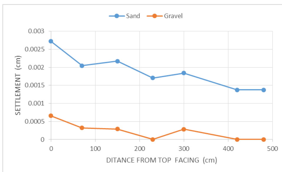
شکل ۴-۸: مقایسه نشست شیروانی برای دو مدل مسلح (پر شده با ماسه و شن)
