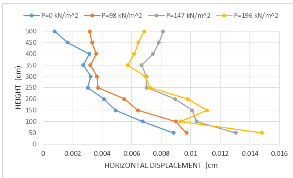
۴-۴۰: مقایسه تغییر مکان افقی نما برای مدل‌های مسلح شده در نما با لایه ژئوسل به طول ۳ متر و با M=200 \text{ kN/m} و پر شده با خاک شن (تأثیر سربار)
