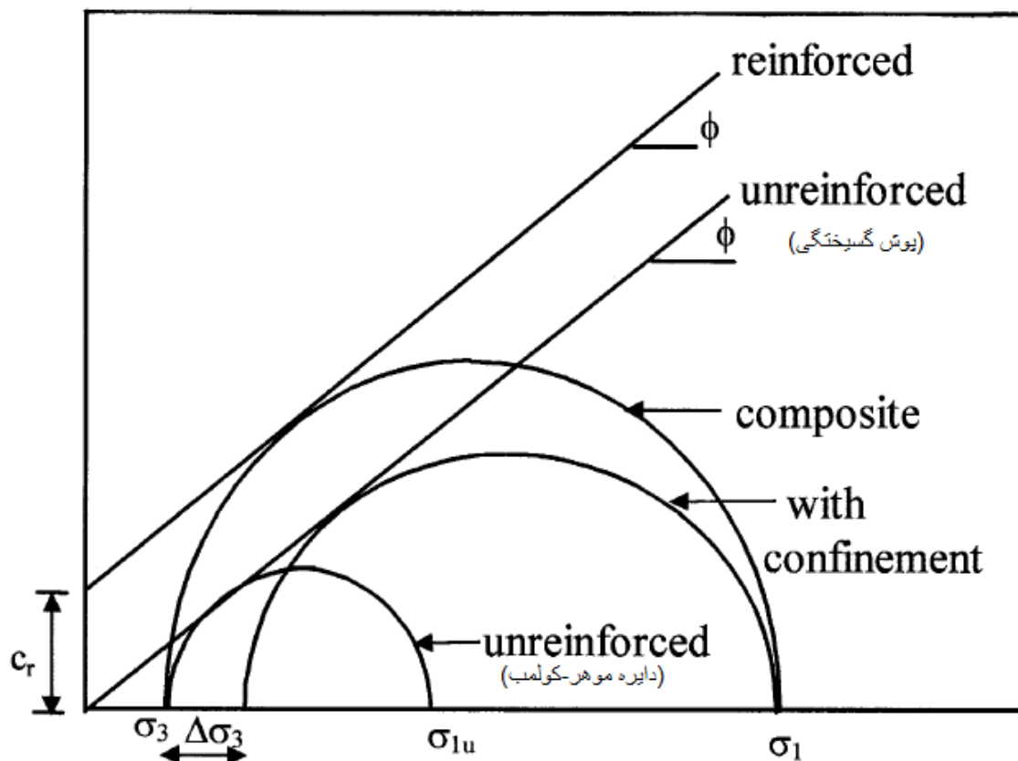
شکل ۲-۲: مقایسه پوش گسیختگی خاک مسلح به ژئوسل و خاک غیرمسلح [10]
