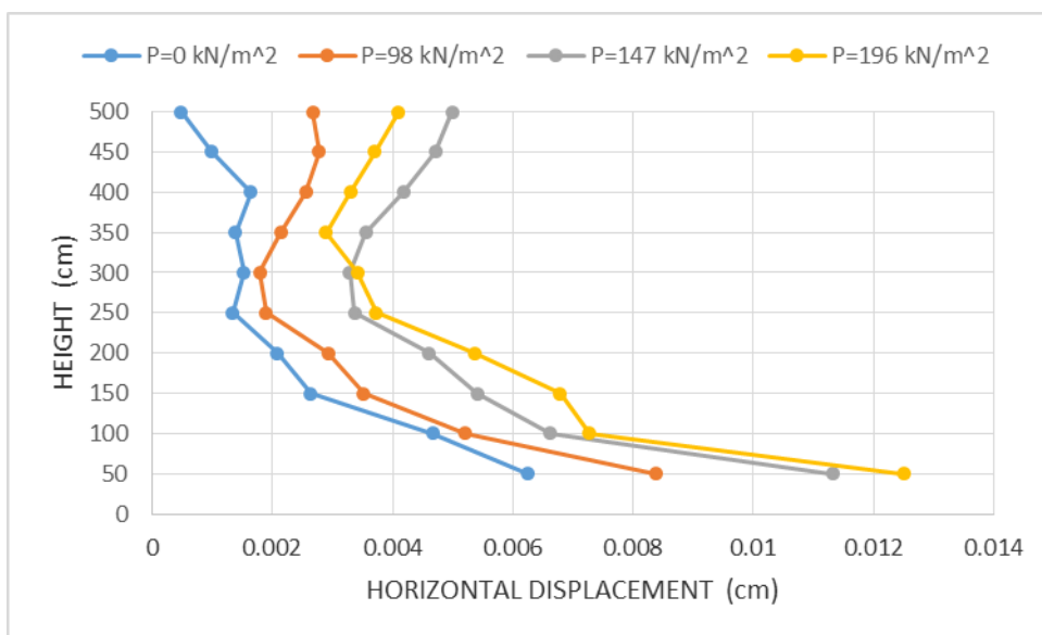
۴-۲۴: مقایسه تغییر مکان افقی نما برای مدل‌های مسلح شده در نما با لایه ژئوسل به طول ۳ متر و با M=500 \text{ kN/m} و پر شده با خاک شن (تأثیر سربار)
