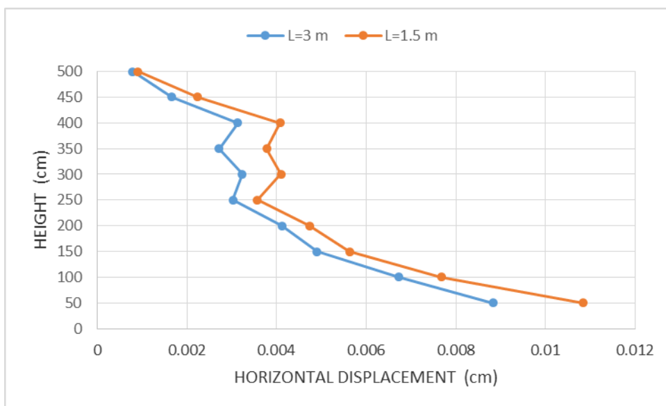
۲۴-۴: مقایسه تغییر مکان افقی نما برای دو مدل مسلح شده در نما با لایه‌های مسلح کننده به طول ۳ و ۱/۵ متر (سلول‌های ژئوسل پر شده با خاک شن و ژئوسل با M=200 \text{ kN/m} )
