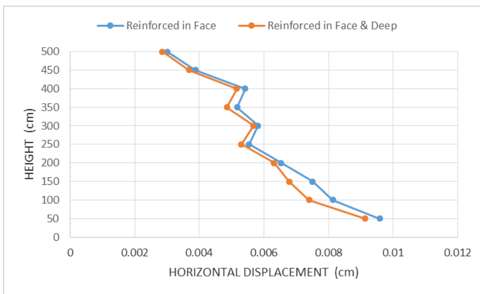
۴-۱۴: مقایسه تغییر مکان افقی نما برای دو مدل مسلح شده در نما و مسلح شده در عمق و نما (سلول‌های ژئوسل پر شده با خاک ماسه ای و ژئوسل با M=200 \text{ kN/m} )
