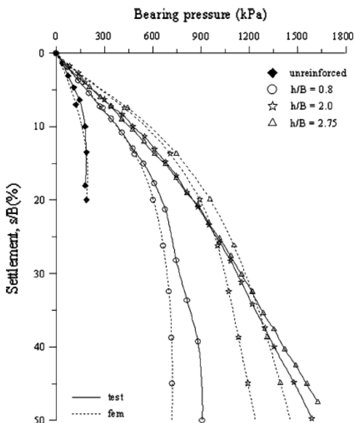
شکل ۲-۳: صحت سنجی استفاده از مدل کامپوزیت جهت مدل‌سازی خاک مسلح به ژئوسل [14]
