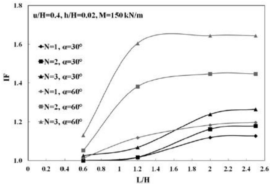
شکل ۲-۱۷: تأثیر طول لایه مسلح کننده برای خاک رسی در پژوهش مهدی پور و همکاران (۲۰۱۳)
