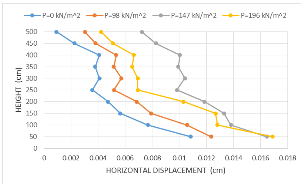
۵۶-۴: مقایسه تغییر مکان افقی نما برای مدل‌های مسلح شده در نما با لایه ژئوسل به طول ۱/۵ متر و با M=200 \text{ kN/m} و پر شده با خاک شن (تأثیر سربار)
