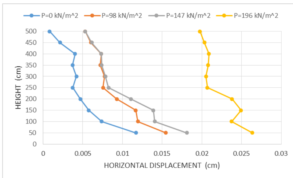
۶۴-۴: مقایسه تغییر مکان افقی نما برای مدل‌های مسلح شده در نما با لایه ژئوسل به طول ۱/۵ متر در نما و ۴ متر در عمق و با M=200 \text{ kN/m} و پر شده با خاک شن (تأثیر سربار)
