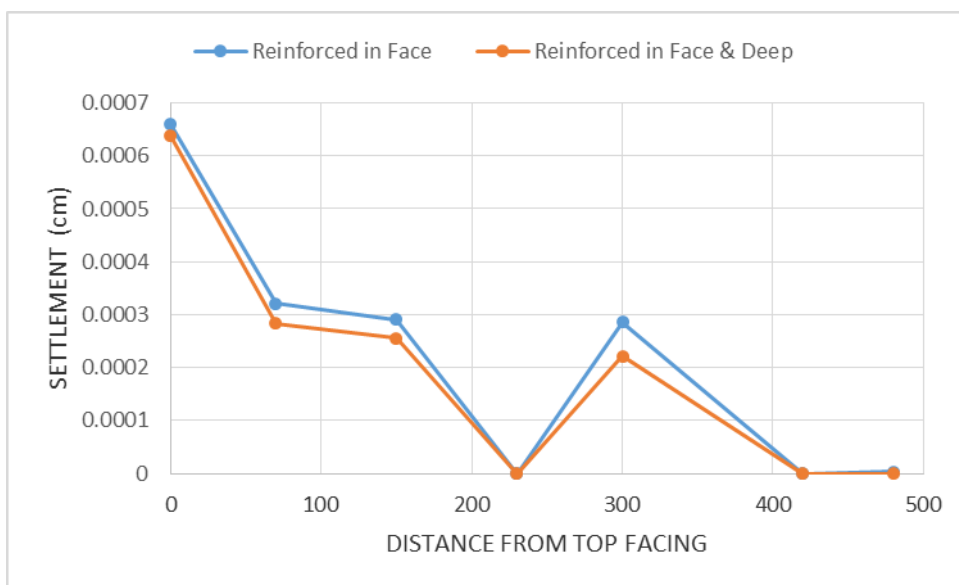
۴-۱۷: مقایسه نشست شیروانی برای دو مدل مسلح شده در نما و مسلح شده در عمق و نما (سلول‌های ژئوسل پر شده با خاک شن و ژئوسل با M=200 \text{ kN/m} )
