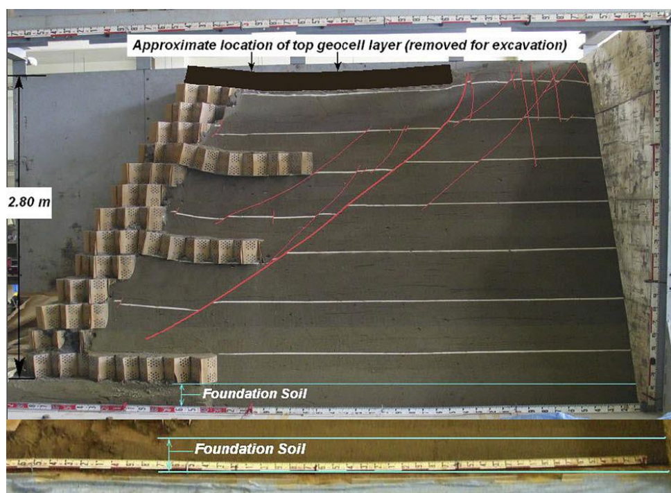
شکل ۲-۲۲: سطوح گسیختگی به وجود آمده در آزمایش چهارم لشچینسکی و همکاران در سال
