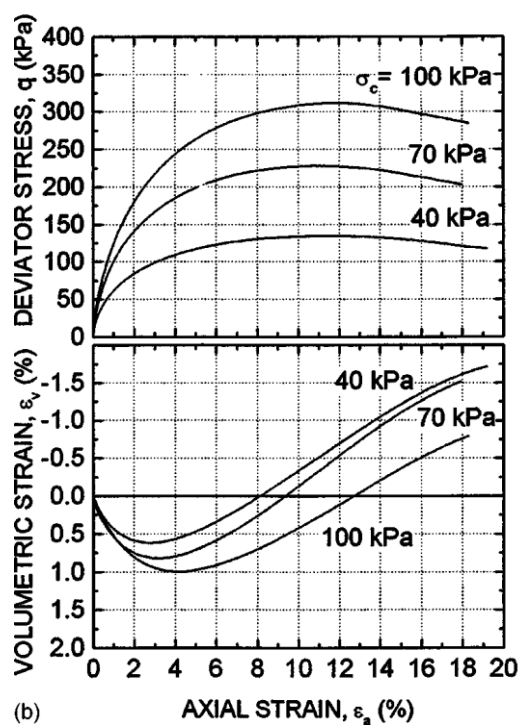
شکل ۳-۲: نتایج آزمایش سه محوری خاک ماسه‌ای لینگ و همکاران (۲۰۰۹) [17]
