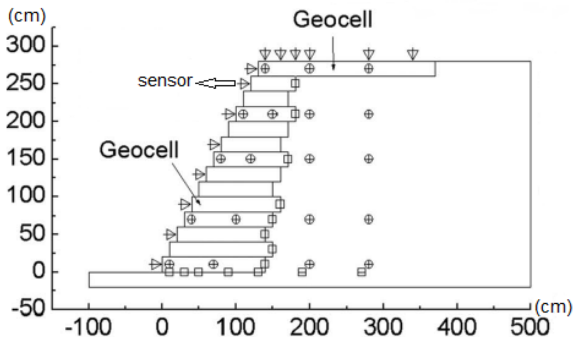
شکل ۳-۱: نمای کلی آزمایش لینگ و همکاران (۲۰۰۹) [17]
