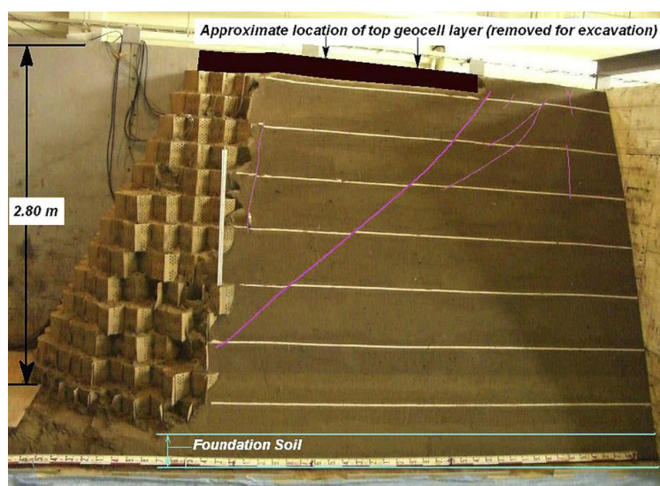
شکل ۲-۲۱: سطوح گسیختگی به وجود آمده در آزمایش سوم لشچینسکی و همکاران در سال
