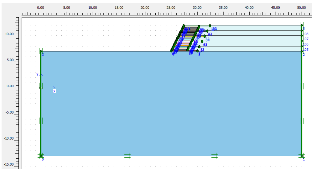
۴-۱۳: نمای کلی از مدل شیروانی و پی آن به همراه لایه‌های افقی ژئوسل در نما و عمق شیروانی
