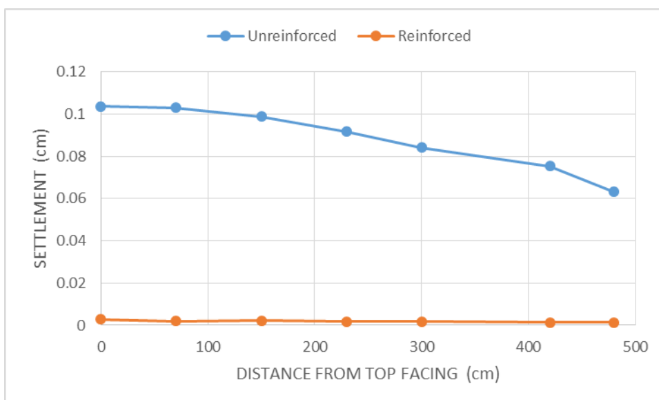
شکل ۴-۳: مقایسه نشست شیب‌ها برای دو مدل غیر مسلح و مسلح
