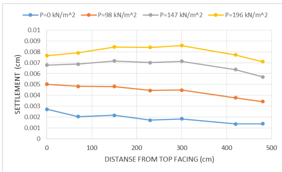
۴-۳۹: مقایسه نشست شیروانی برای مدل‌های مسلح شده در نما با لایه ژئوسل به طول ۳ متر و با M=200 \text{ kN/m} و پر شده با خاک ماسه (تأثیر سربار)
