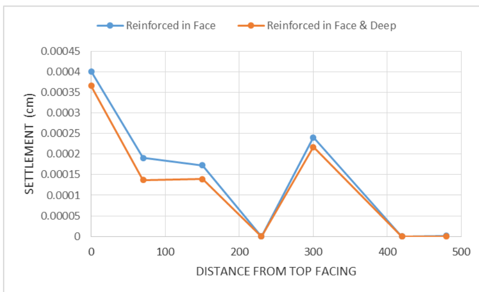
۲۱-۴: مقایسه نشست شیروانی برای دو مدل مسلح شده در نما و مسلح شده در عمق و نما (سلول‌های ژئوسل پر شده با خاک شن و ژئوسل با M=500 \text{ kN/m} )
