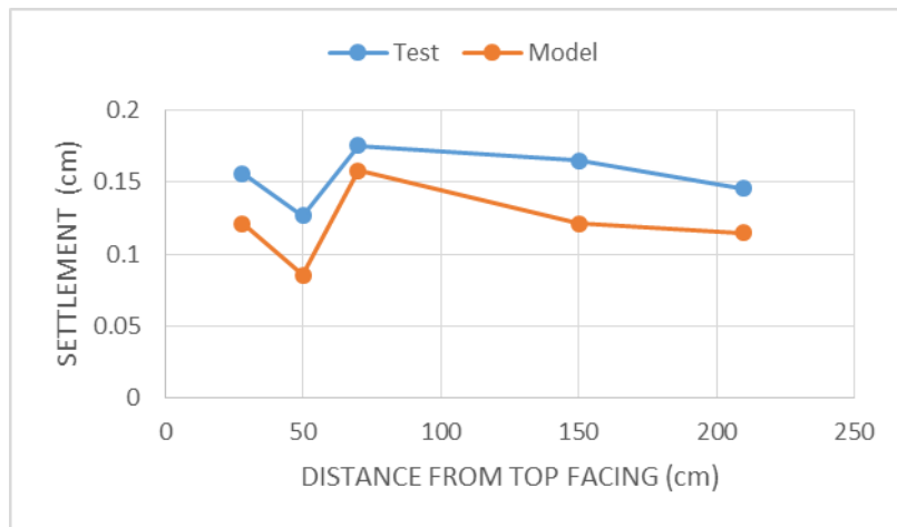
شکل ۳-۱۰: مقایسه نشست بالای دیوار در آزمایش و مدل‌سازی
