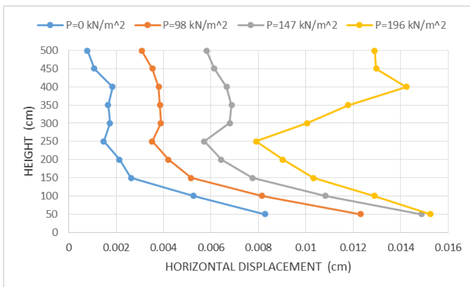
۶۰-۴: مقایسه تغییر مکان افقی نما برای مدل‌های مسلح شده در نما با لایه ژئوسل به طول ۱/۵ متر و با M=500 \text{ kN/m} و پر شده با خاک شن (تأثیر سربار)
