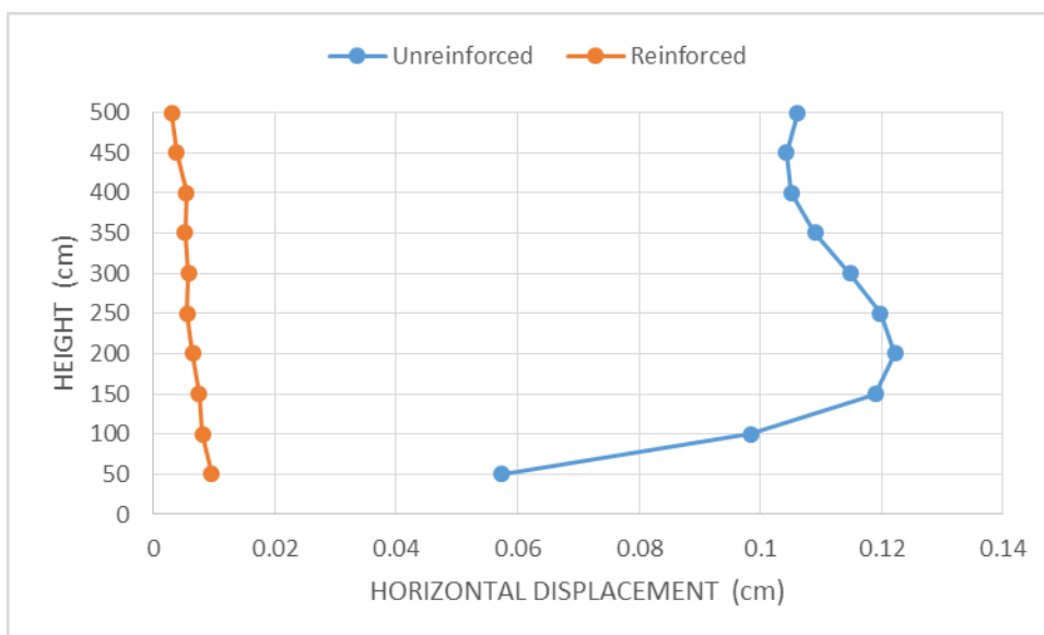
شکل ۴-۲: مقایسه حداکثر جابه‌جایی افقی نما برای دو مدل غیر مسلح و مسلح
