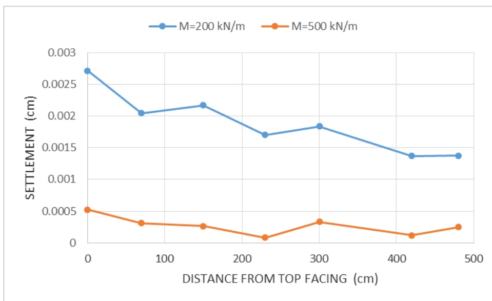
۴-۱۰: مقایسه نشست شیروانی برای دو مدل مسلح شده با ژئوسل با سختی محوری ۲۰۰ و ۵۰۰ کیلونیوتن برمتر (پوشده با ماسه)
