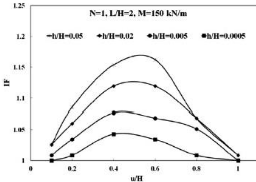
شکل ۲-۱۸: تأثیر ضخامت لایه مسلح کننده برای خاک ماسه‌ای در پژوهش مهدی پور و همکاران [۲۰۱۳] [15]
