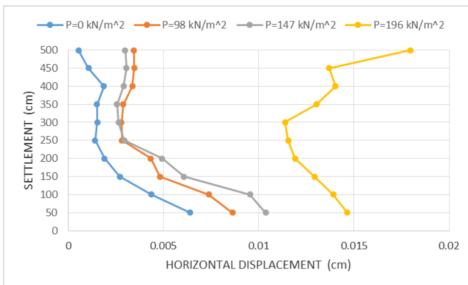
۴-۵۰: مقایسه تغییر مکان افقی نما برای مدل‌های مسلح شده در نما با لایه ژئوسل به طول ۳ متر در نما و ۵ متر در عمق و با M=500 \text{ kN/m} و پر شده با خاک ماسه (تأثیر سربار)
