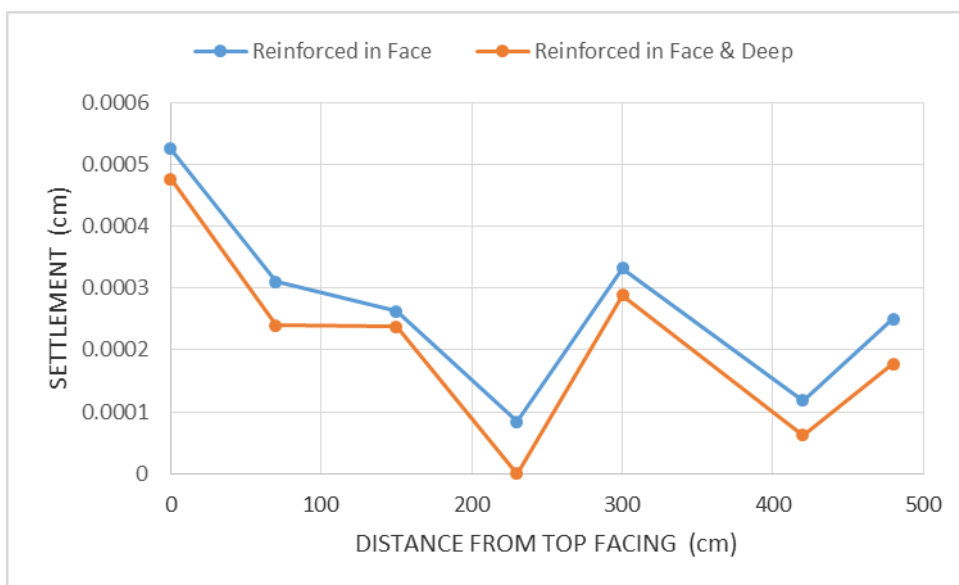
۴-۱۹: مقایسه نشست شیروانی برای دو مدل مسلح شده در نما و مسلح شده در عمق و نما (سلول‌های ژئوسل پر شده با خاک ماسه و ژئوسل با M=500 \text{ kN/m} )
